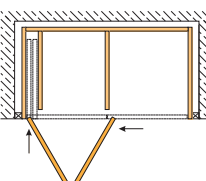
montážní schéma pro vložené dveře umístěné v nice
