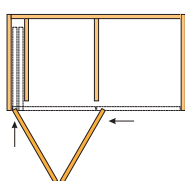
montážní schéma pro vložené dveře s bočnicemi
