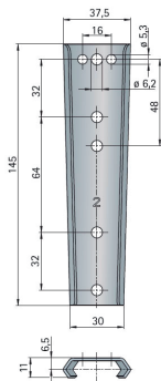
Zástrčné spojovací kování 2 1.20.420.02.05
